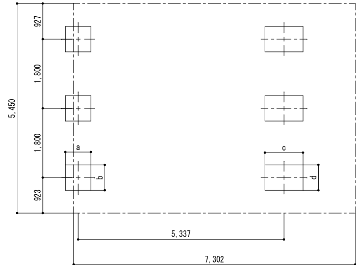
■ 基礎配置図
